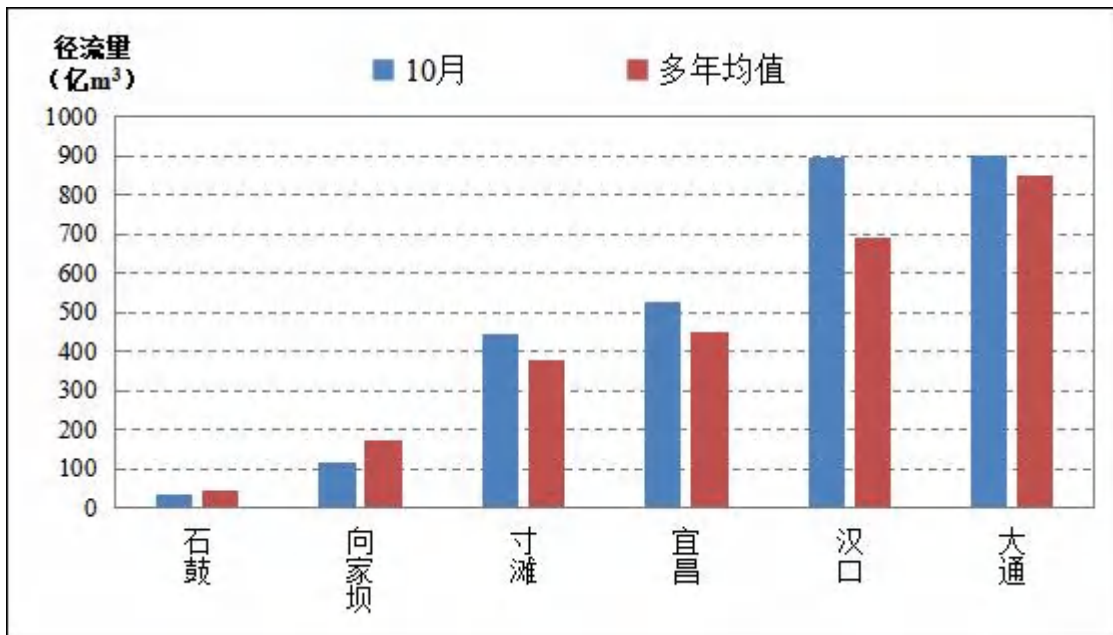
图 1-1 2025 年 10 月长江干流主要控制站径流量与多年均值对比
