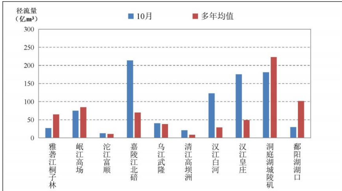
图 1-2 2025 年 10 月长江流域重要水系节点控制站径流量与多年均值对比
