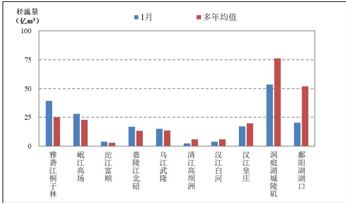
图 1-2 2025 年 1 月长江流域重要水系节点控制站径流量与多年均值对比
