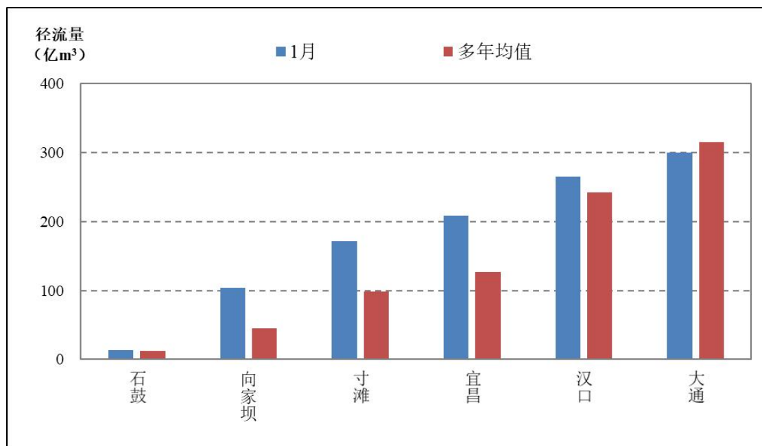
图 1-1 2025 年 1 月长江干流主要控制站径流量与多年均值对比
